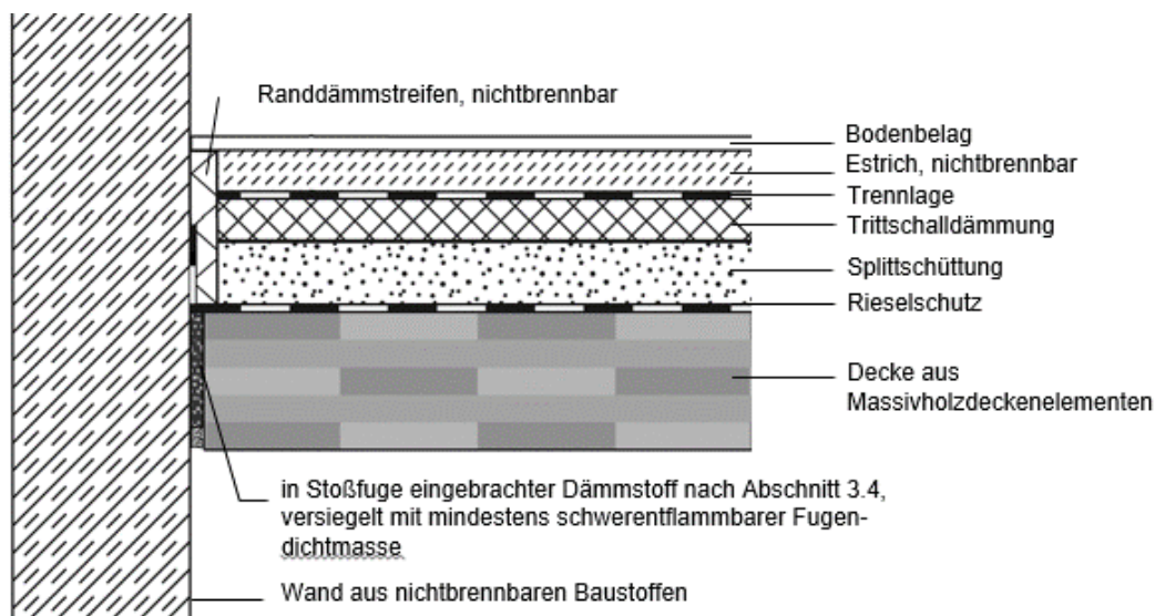
Prinzipskizze 10: Bauteilanschluss unbekleidete Massivholzdecke / Wand aus nichtbrennbaren Baustoffen (Vertikalschnitt)
