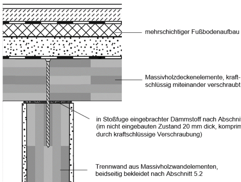
Prinzipskizze 8c: Anschluss Trennwand / Massivholzdecke, Bauteilfuge (Vertikalschnitt)
