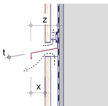
Prinzipskizze 14: Ausführung und Befestigung von horizontalen Brandsperrn
