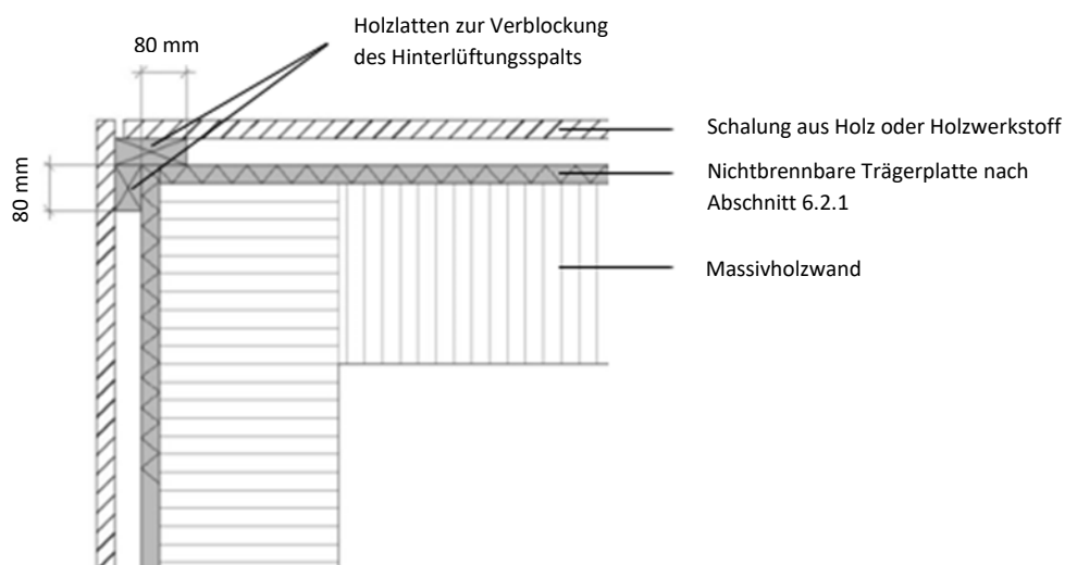
Prinzipskizze 13: Ausbildung Außenwandbekleidung bei Außenecken (Horizontalschnitt)
