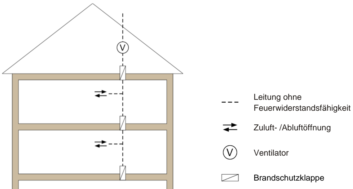
Bild 2.1: Schottlösung
