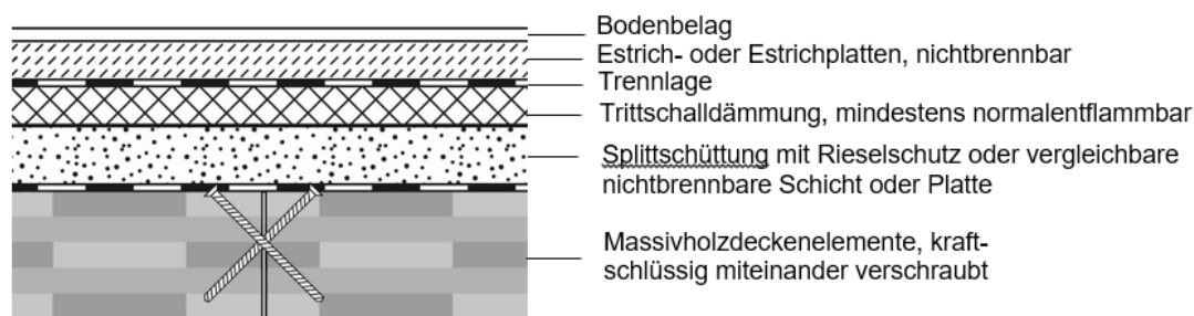
Prinzipskizze 7: unbelagte Massivholzdecke mit verschraubter Elementfuge und mehrschichtigem, hohlraumfreiem Fußbodenaufbau (Vertikalschnitt)
