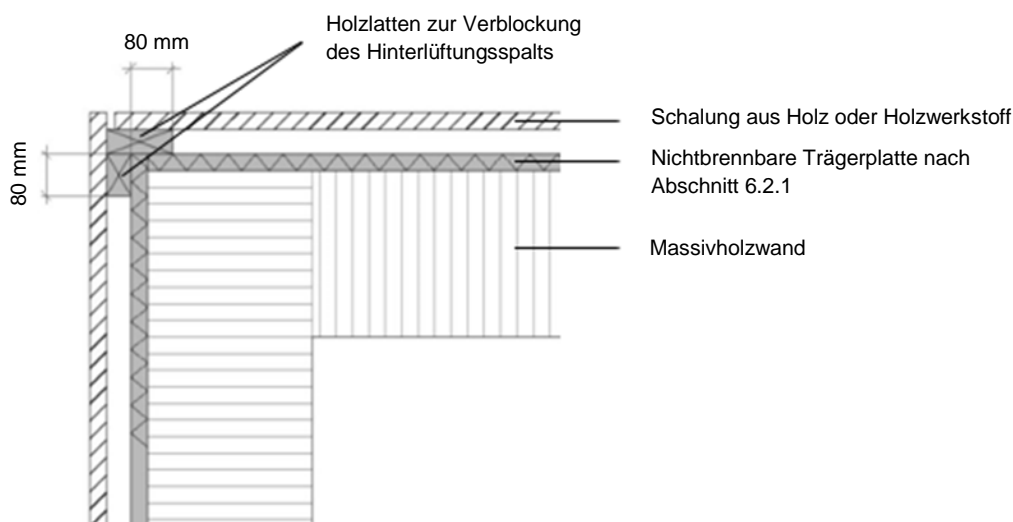
Prinzipskizze 13: Ausbildung Außenwandbekleidung bei Außenecken (Horizontalschnitt)
