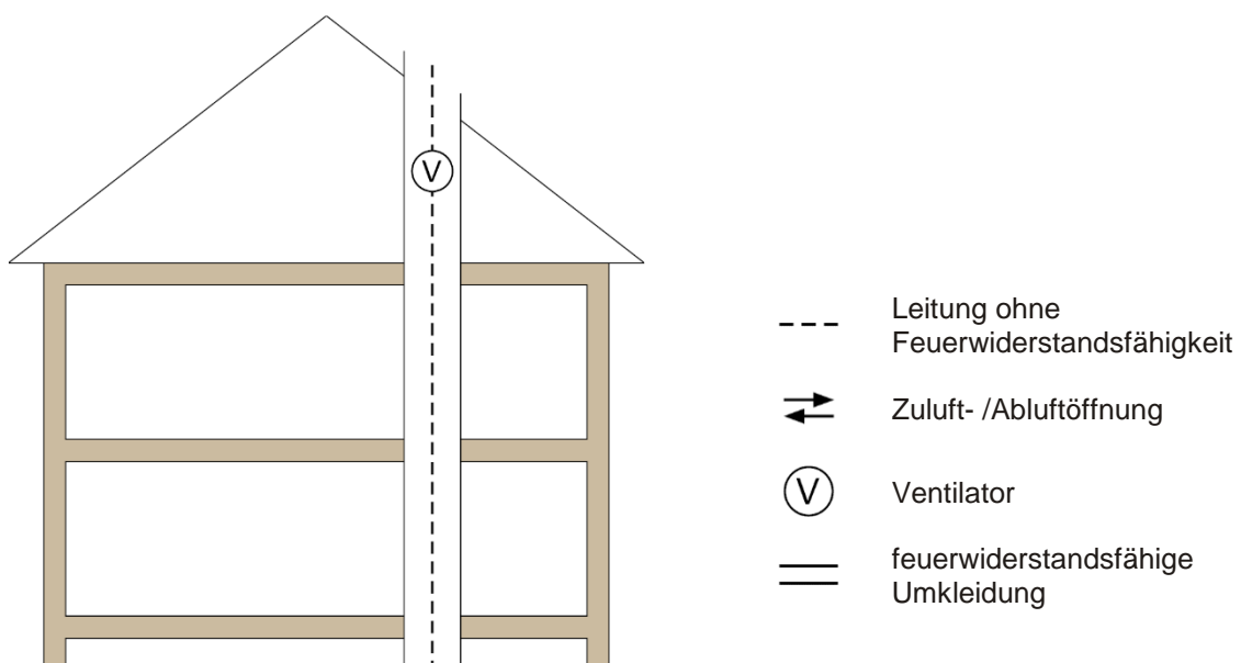
Bild 2.2: Schachtlösung
