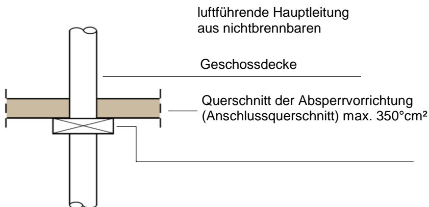
Bild 6.2: Beispiel für Schottlösung für Lüftungsanlagen nach DIN 18017-3:2009-09 maximaler Anschlussquerschnitt der Absperrvorrichtungen: 350 cm 2
