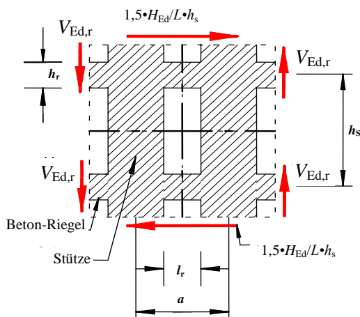
Abb. 2: Bezeichnungen
