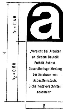
Bild 1: Kennzeichnung
