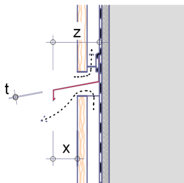
Prinzipskizze 14: Ausführung und Befestigung von horizontalen Brandsperrern
