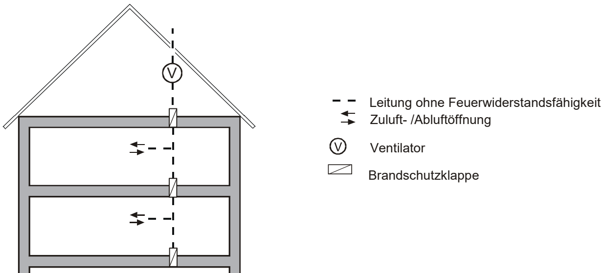
Bild 2.2: Schachtlösung
