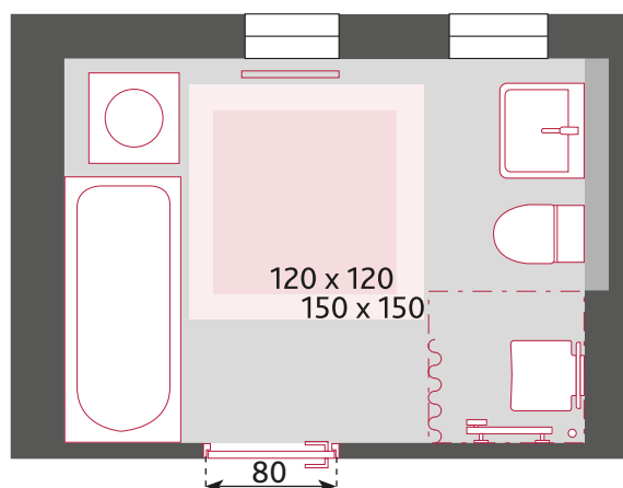
Umbau barrierefrei nach DIN 18040-2
