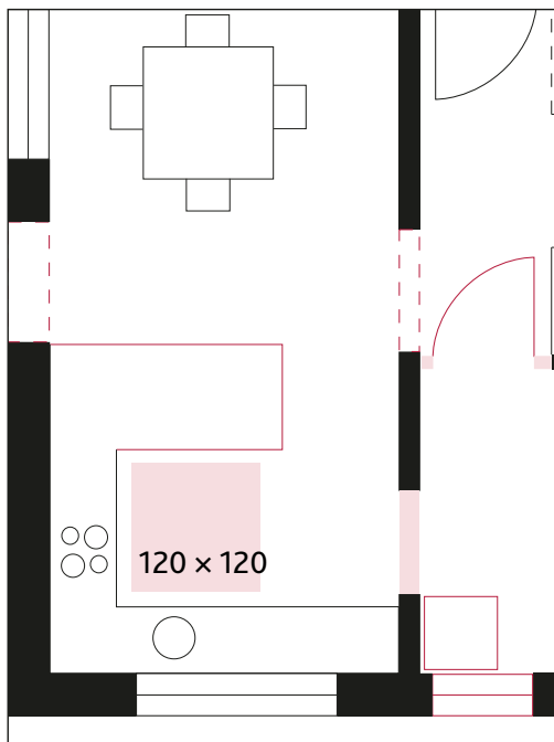
64 – 65 U- und L-förmige Küchen mit integrierten bzw. angelagerten Essplätzen
