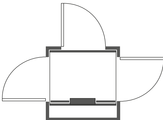
46 Exemplarischer Grundriss Senkrechtlift – Türen an bis zu drei Seiten möglich
