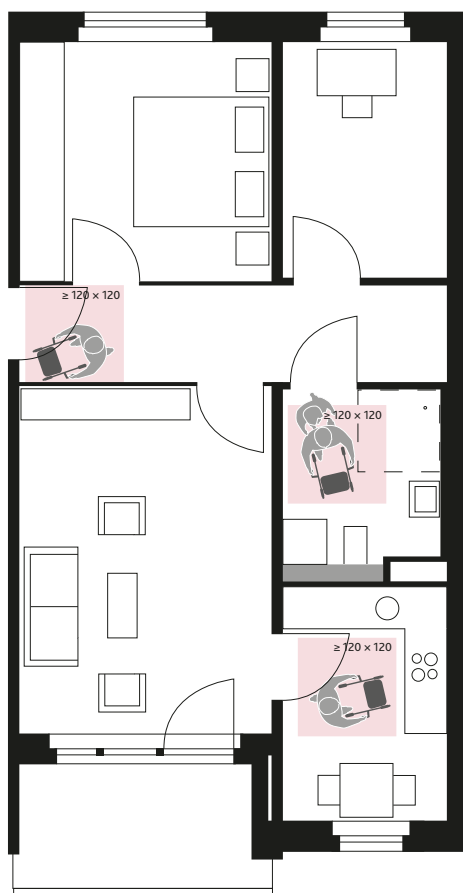
Grundriss nach Umbau
