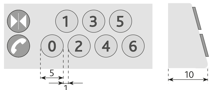
40 Geneigtes Bedientableau nach DIN EN 81-70 (Anhang G) mit Befehlsgebern Typ XL
