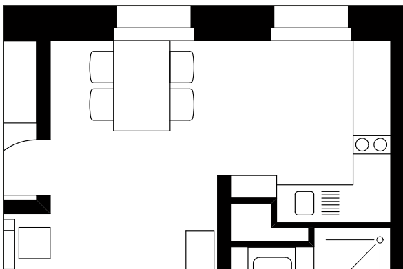
66 – 67 L-förmige Küchen mit angelagerten Essplätzen; Am Weidenschlag, GAG Ludwigshafen
