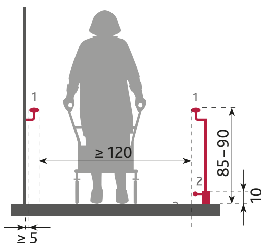
18 Rampe, Querschnitt 1 Handlauf; 2 Holm als Radabweiser
