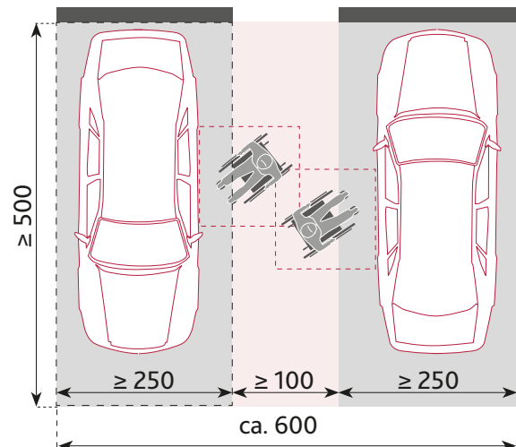
25 Barrierefreie Stellplätze mit gemeinsam genutzter Bewegungsfläche und Grundabmessung nach DIN 18040 (350 × 500 cm)
