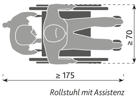
5 Maße verschiedener Hilfsmittel
