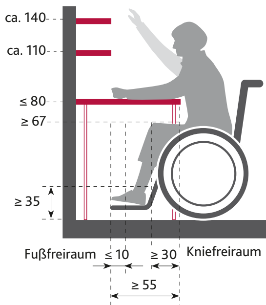
68 Greifhöhen und Unterfahrbarkeit für Rollstuhlfahrerinnen und -fahrer
