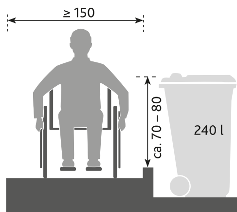
22 Höhenversetzte Gestaltung für große Müllbehälter
