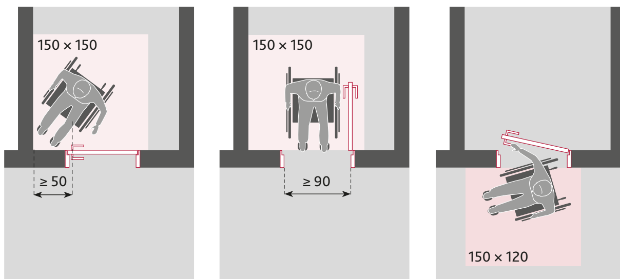
27 Bewegungsablauf und Bewegungsflächen bei Drehflügeltüren nach DIN 18040-2
