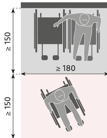
3 Platzbedarf beim Umsetzen vom Straßen- auf den Zimmerrollstuhl
