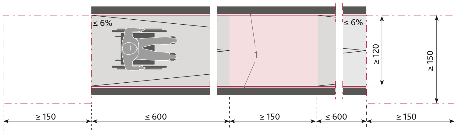
19 Grundriss Rampe nach DIN 18040-2
