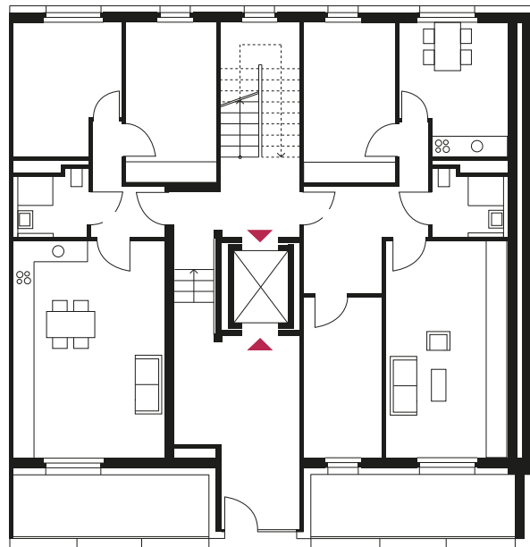
47 Grundriss EG mit Aufzug nach Umbau, Gartenstadt Drewitz, Potsdam
