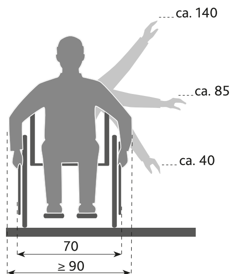
29 Greif- und Bedienhöhen für Rollstuhlfahrerinnen und -fahrer
