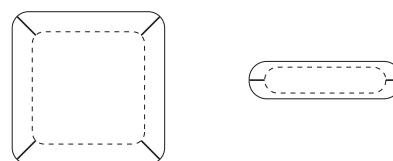
36 Greifgünstige Ausbildung von Handläufen; aus: Leitfaden Barrierefreies Bauen (s. Quellenverzeichnis 12)
