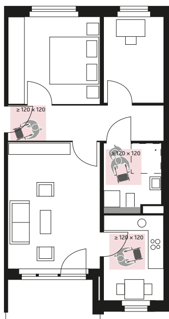
Bewegungsflächen von 120 x 120 cm
