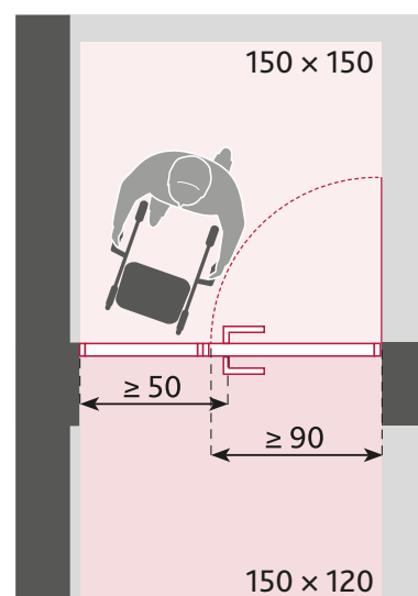
26 Bewegungsflächen an Hauseingangstüren gemäß DIN 18040-2
