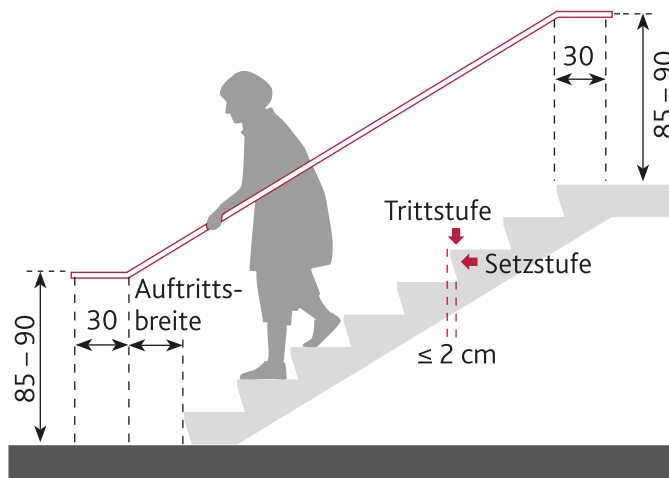
35 Anforderungen an Treppen und Handläufe gemäß DIN 18040-2; schräge Setzstufen mit \leq 2 cm Unterschneidung sind zulässig
