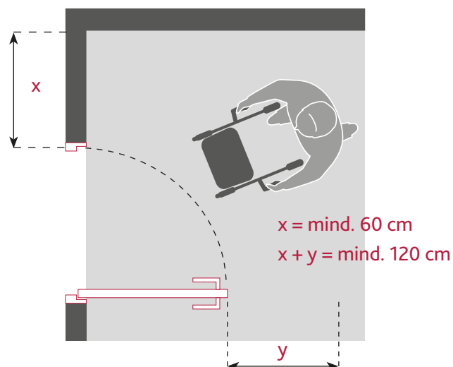
50 Formel zur Berechnung der Bewegungsfläche vor Wohnungstüren nach SIA 500
