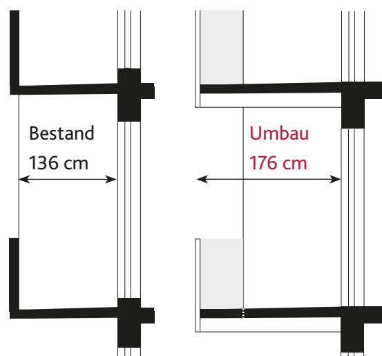
60 Vergrößerung der nutzbaren Tiefe durch Verlängerung Balkon/Loggia.
