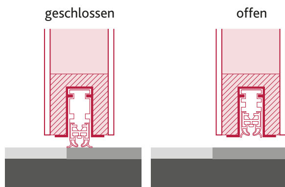
56 Türdichtung, die in geschlossenem Zustand abgesenkt ist
