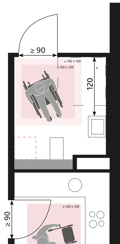
Grundriss Bad Nutzung mit Rollstuhl
